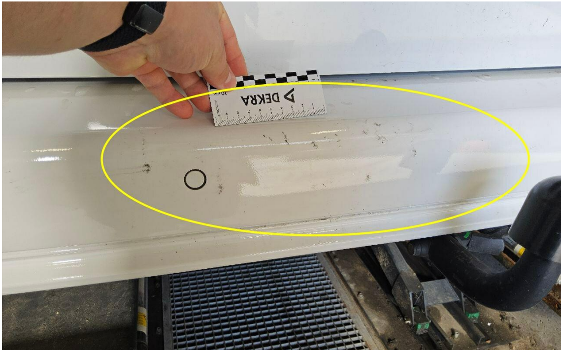
Bild 19 : Stoßfänger hinten, verschrammt
