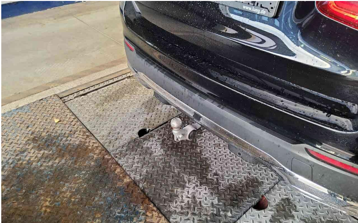
Bild 7 : Kugelkopf bei abnehmbarer AHK
